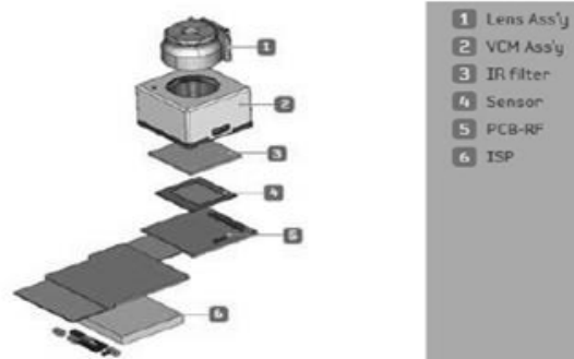
<카메라 모듈 구성도>
