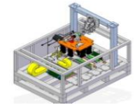
Edge Crack AOI
