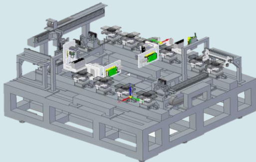
[2차 전지 외관 검사장비]
