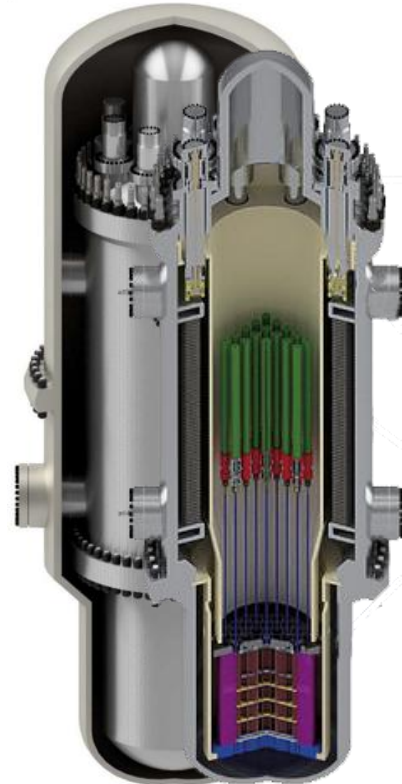
[SMR 내부 구성 및 주요 부품]
